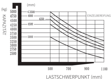
Hublastdiagramm
