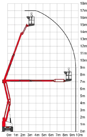
Arbeitsdiagramm
